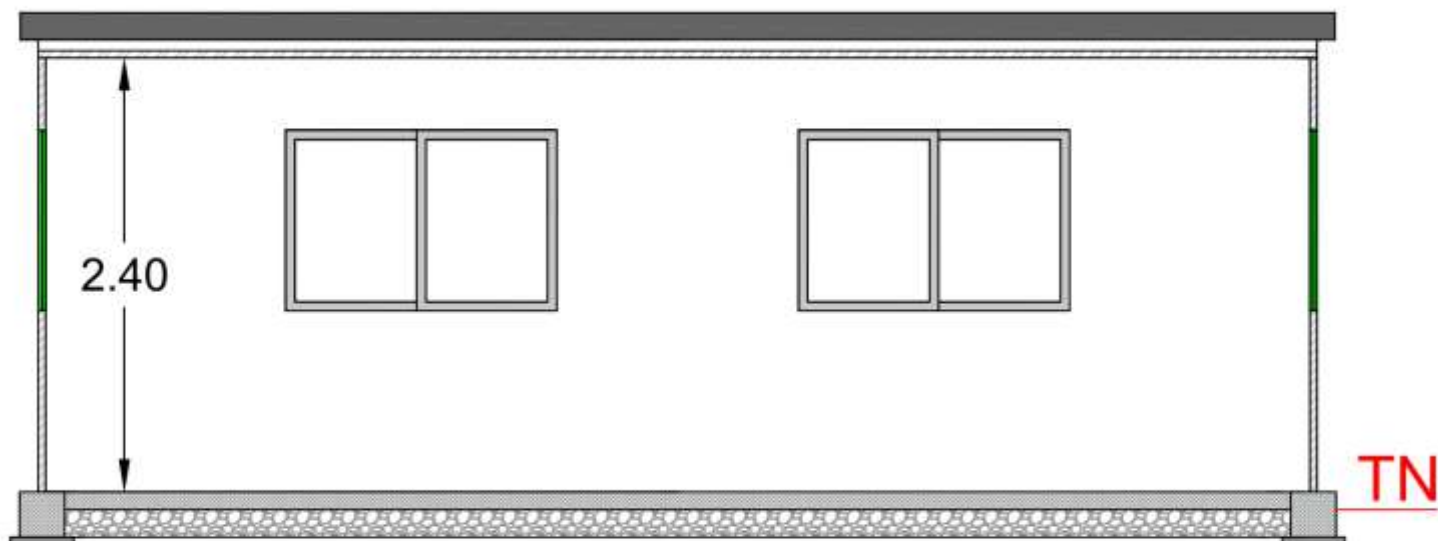
Coupe B-B
