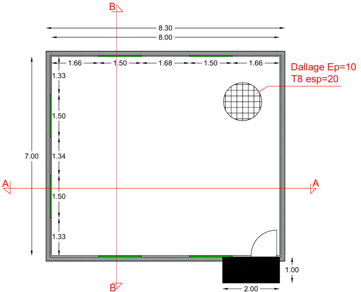
Plan de coffrage et ferrailage du dallage
