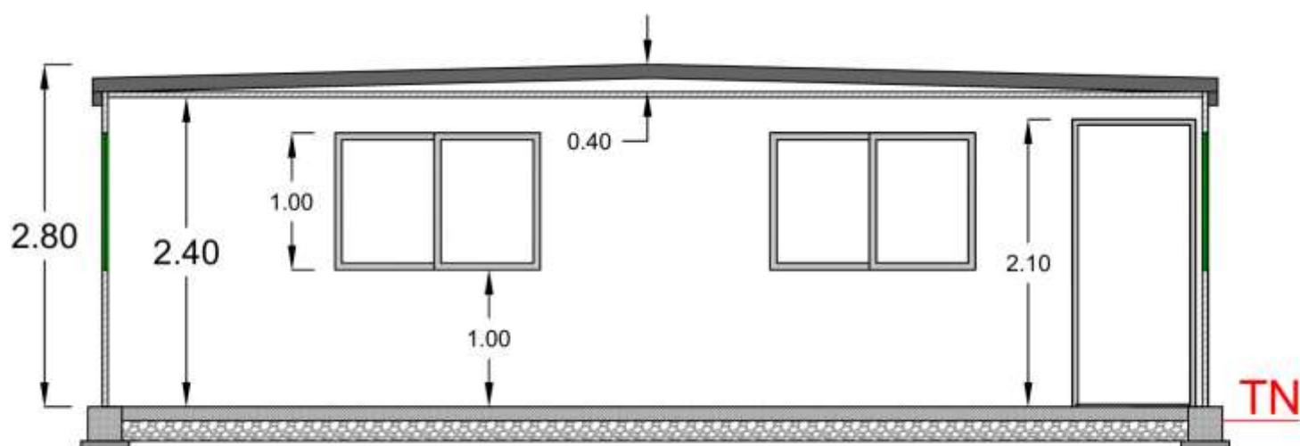
Coupe A-A
