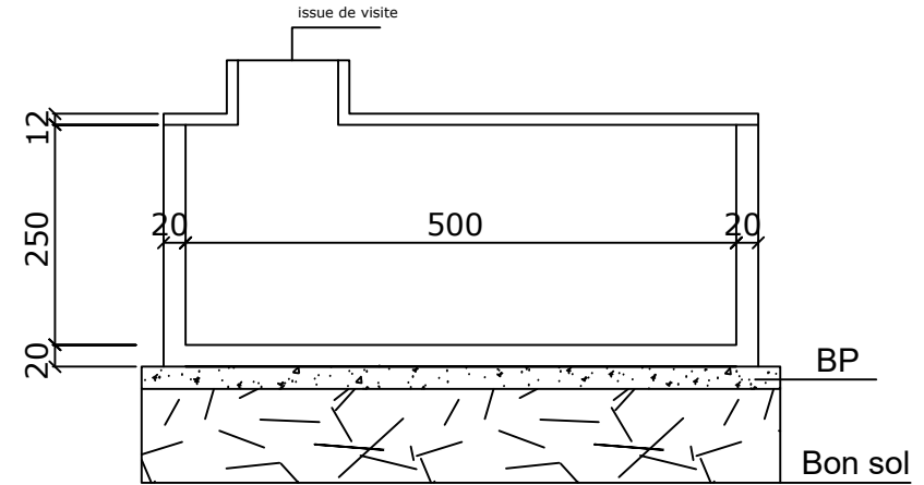
COUPE LONGITUDINALE DE RESERVOIR DE CAPACITE 48m3 soit (5x4x2.5)
