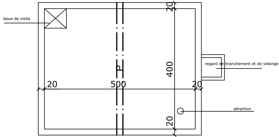
VUE EN PLAN DE RESERVOIR DE CAPACITE 48m3 soit (5x4x2.5)
