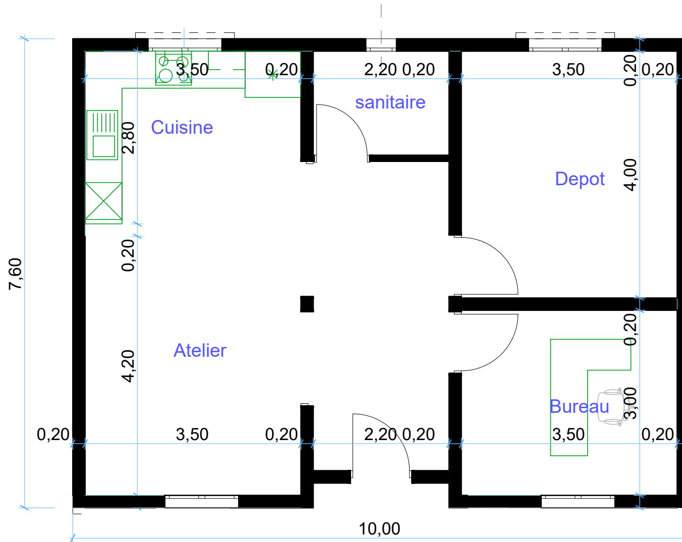
PLAN RDC
